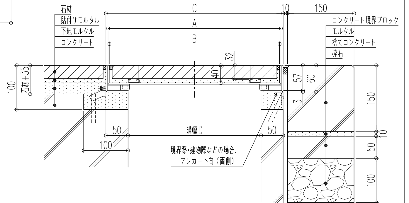
施工参考図
